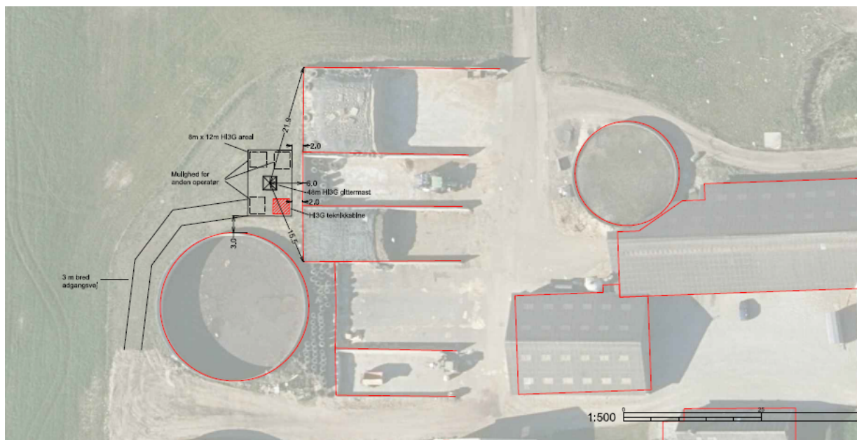
Udsnit af situationsplan der viser hvor masten opsættes
