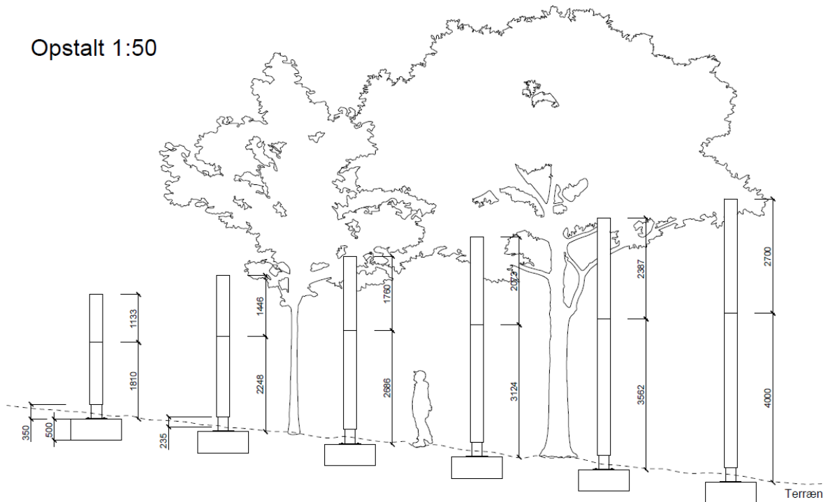
Opstalt af naturkirken
