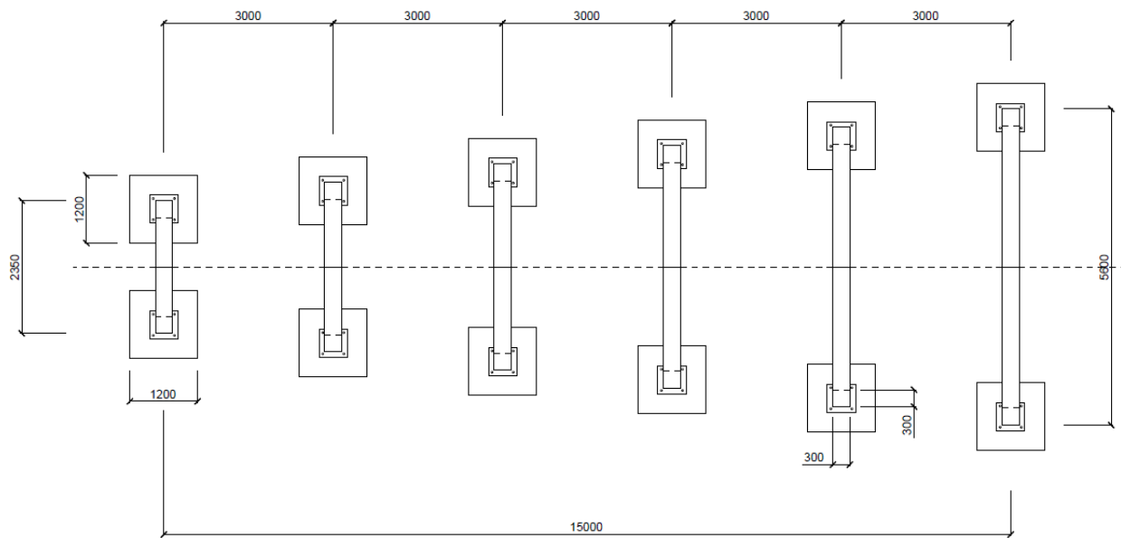
Plantegning af naturkirken
