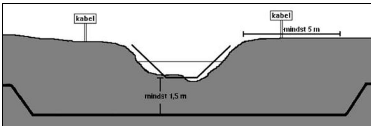
Figur 2: Korrekt kabelunderføring
