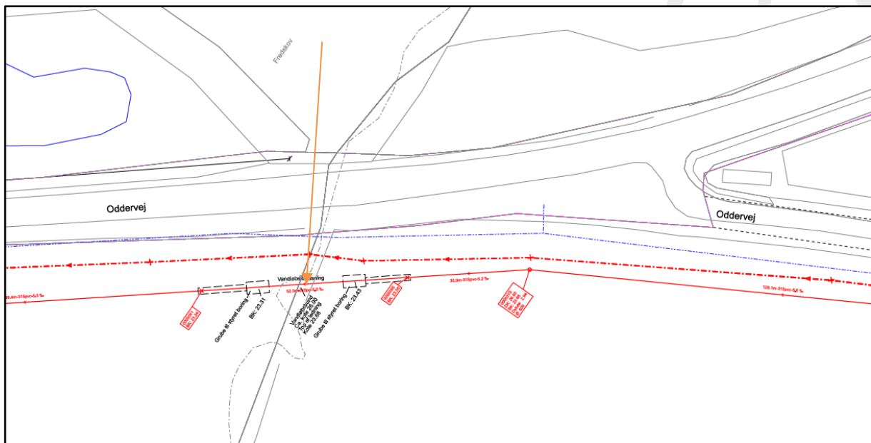
Figur 1: Krydsningspunkt (orange pil) samt boregruber til styret underboring. Rød fuldoptrukket linje illustrerer projekteret spildevandsledning (fra Skanderborg Forsynings ansøgningsmateriale).
