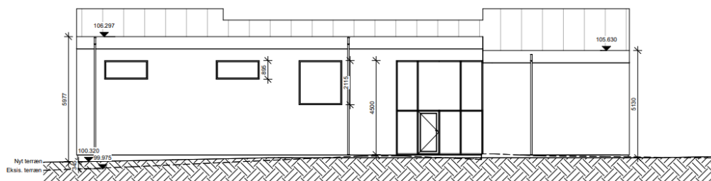
Østfacade (ny) 1 : 100
