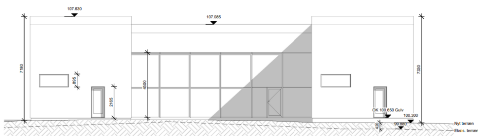
Østfacade (ny) 1 : 100
