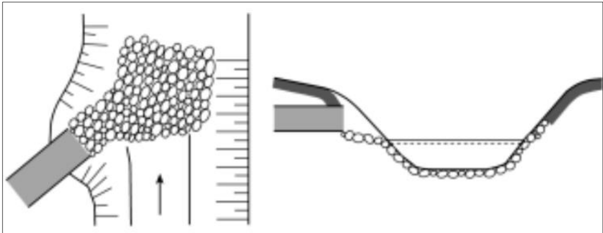
Figur 1. Udløb udformes og placeres så mindst mulig erosion af bund og brinker opnås. Bund og brinker sikres eksempelvis med stensætning.
