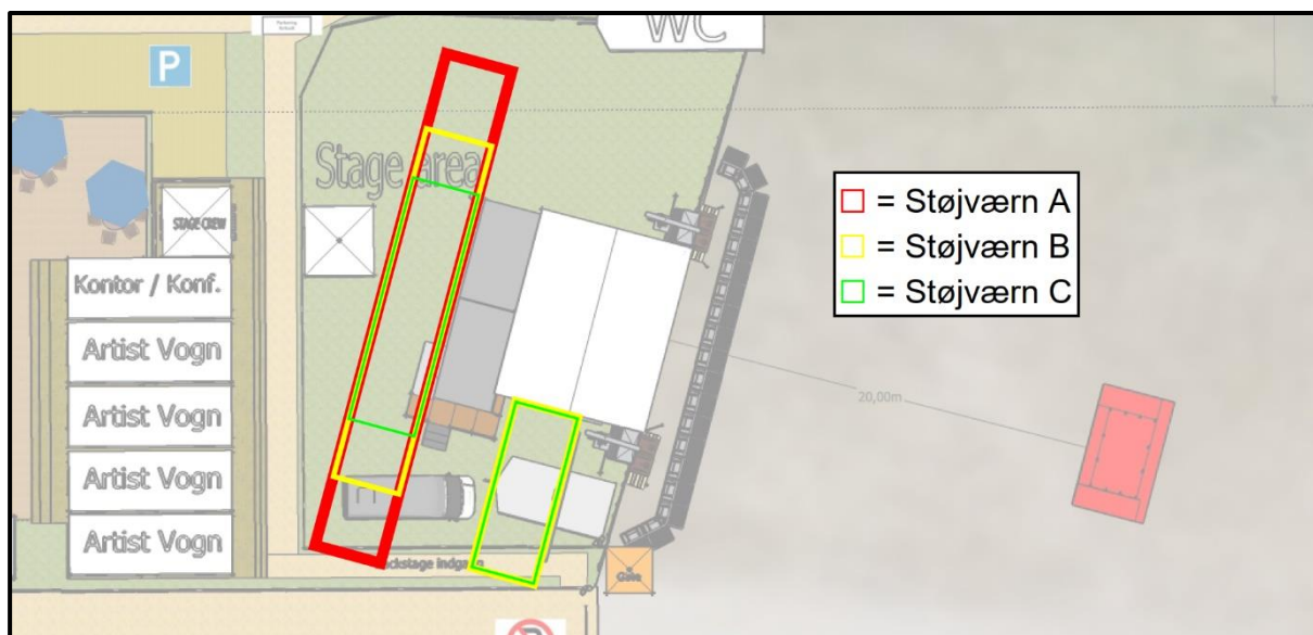
Figur 6.1: Placering af de 3 forskellige beregnede støjværn.
