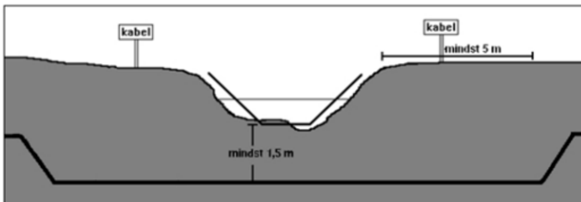
Figur 1. Korrekt kabelføring.
