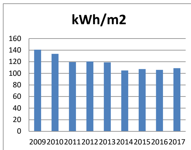
Figur 3. Energiforbrug pr. m 2 kommunal bygning
