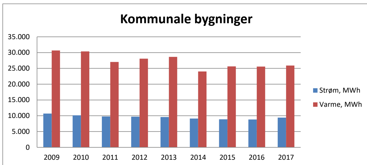
Figur 1. Energiforbrug til hhv. strøm og varme i de kommunale bygninger
