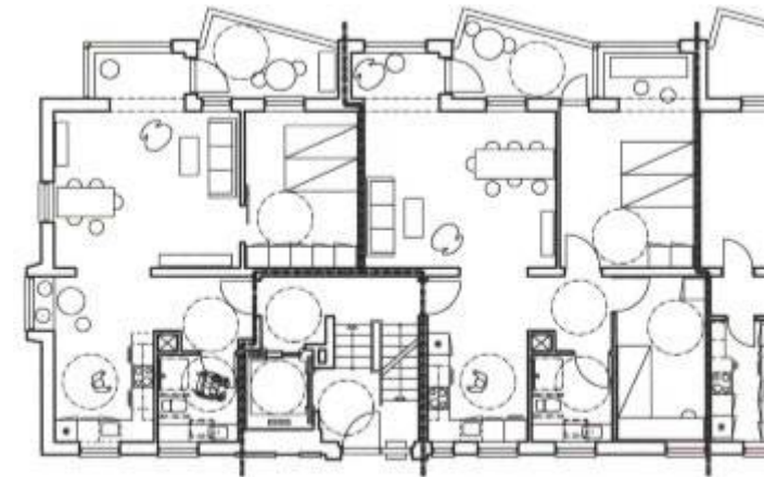
STUEPLAN, 1. OG 2. SAL - FREMTIDIGE FORHOLD 1:150 (A3)
