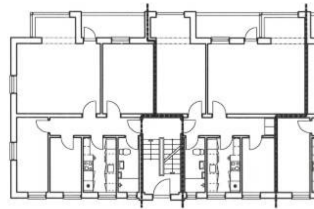
STUEPLAN, 1. OG 2. SAL - EKSISTERENDE FORHOLD 1:150 (A3)
